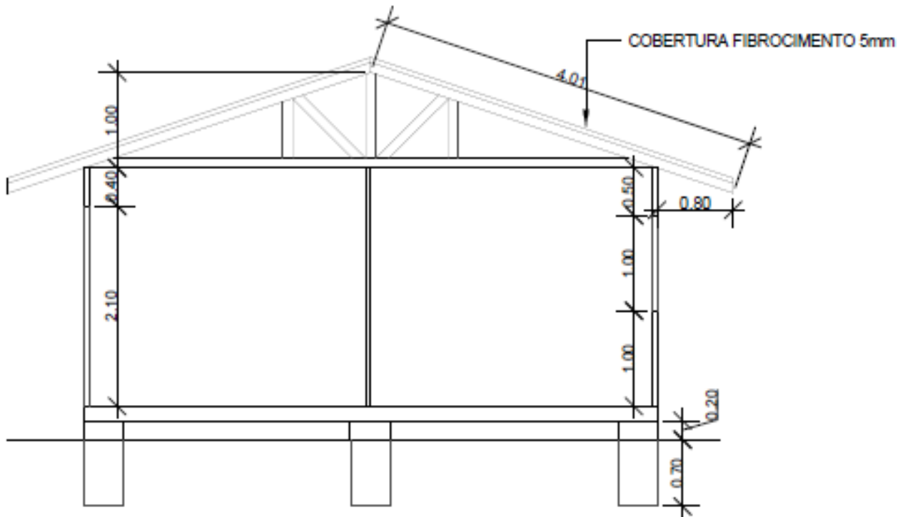
CORTE "A,A"
