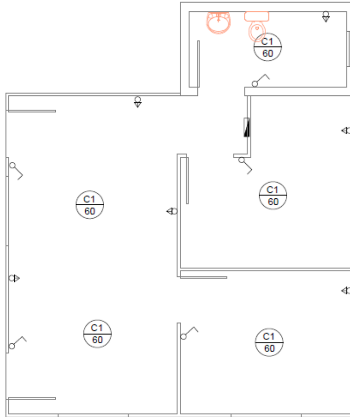
PLANTA ELETRICA
