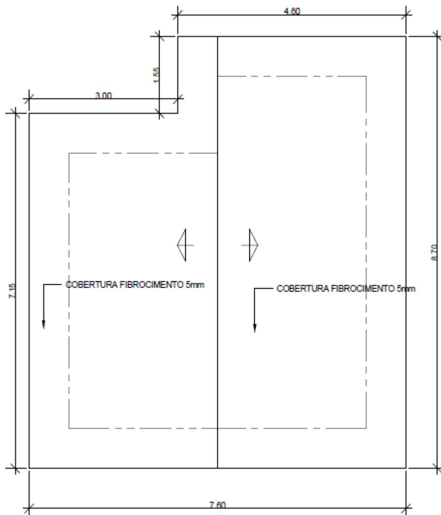
PLANTA DE COBERTURA
